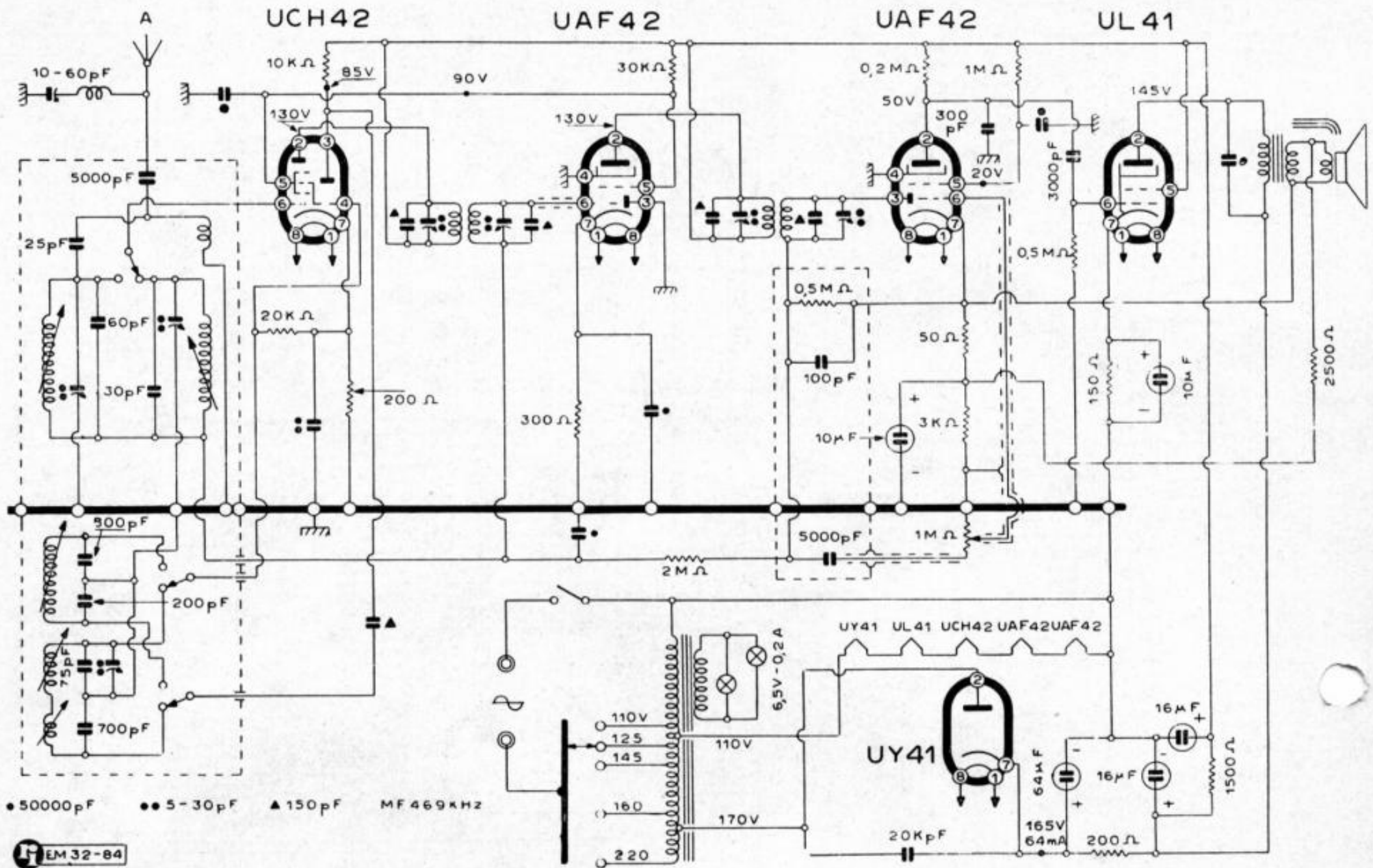
SIEMENS S.A. - Mod. SM 524
